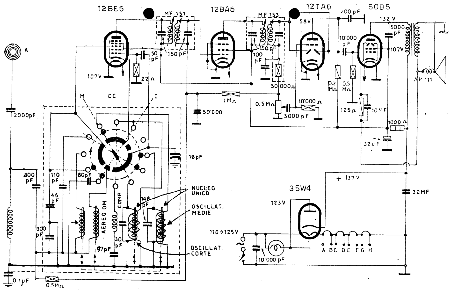
UNDA RADIO - Mod. 53/25 - Media frequenza 467 kc. Massima corrente anodica 75 mA. Massima corrente alternata 250 mA. Per corrente continua o alternata della rete a 110 sino a 127 volt.
